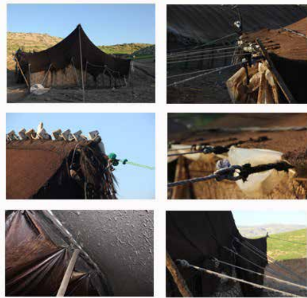
تصویر ۱. اجزای تشکیل دهنده سیاه چادر، مأخذ: نگارندگان، ۱۳۹۷.
